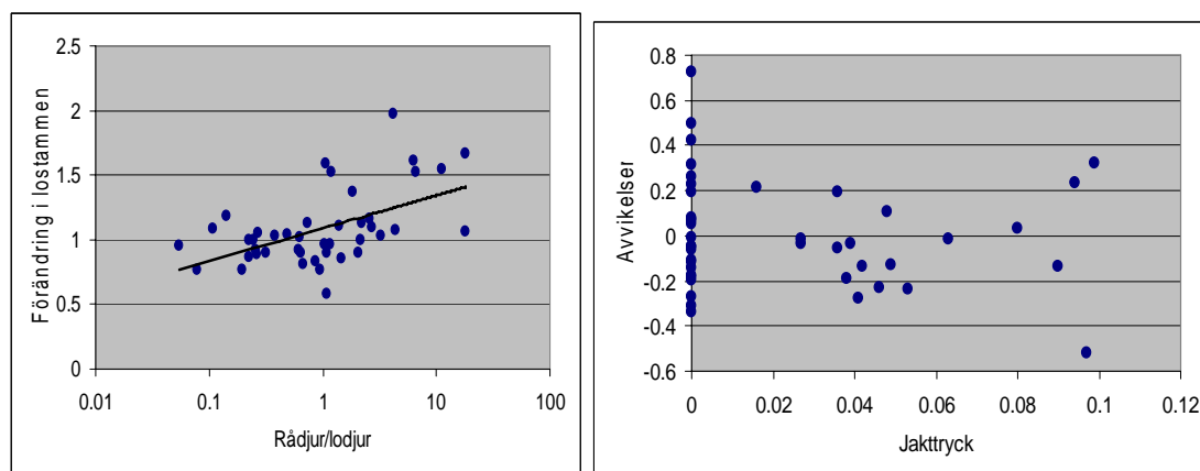
Figur 11. Förändring i lodjursstammen från ett år till nästa ( \lambda ) i relation till kvoten mellan avskjutning av rådjur/tätheten av lofamiljegrupper i Sverige söder om renskötseområdet, samt analys av avvikelserna från förväntad förändring i relation till jakttrycket.
